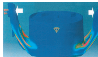
Rotor classique mis sous pression
